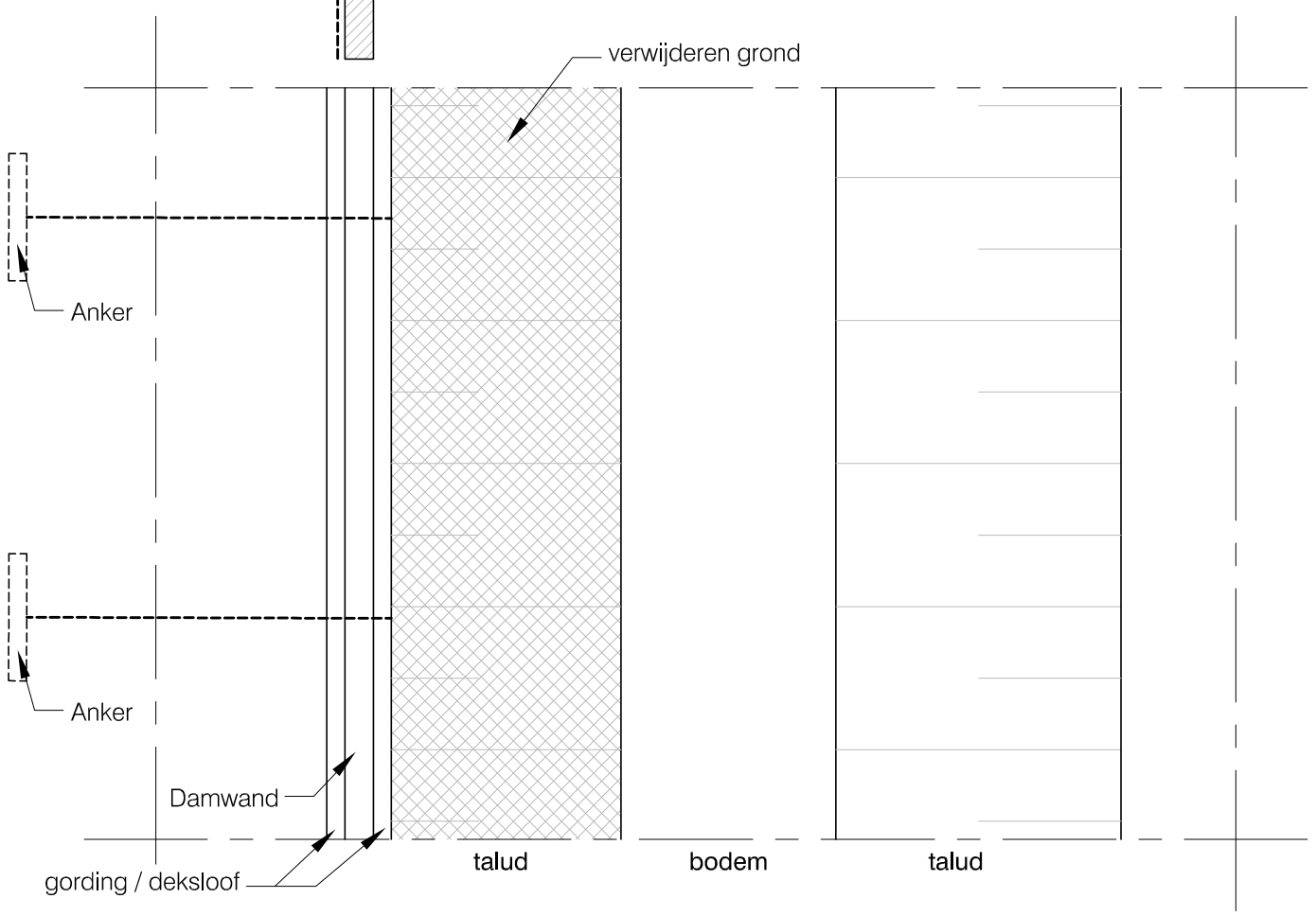
Bovenaanzicht
